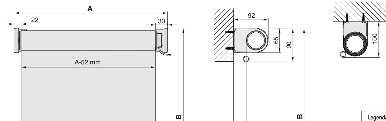
APOLLO PLUS - motor
