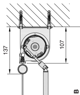
V63 - klika s vedením, montáž na strop
