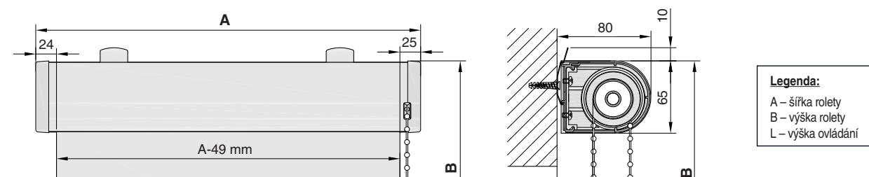
MODULA 36 - PK (s montážním Profilem a Kazetou)
