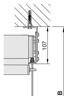
V63 - klika s vedením, montáž na strop
