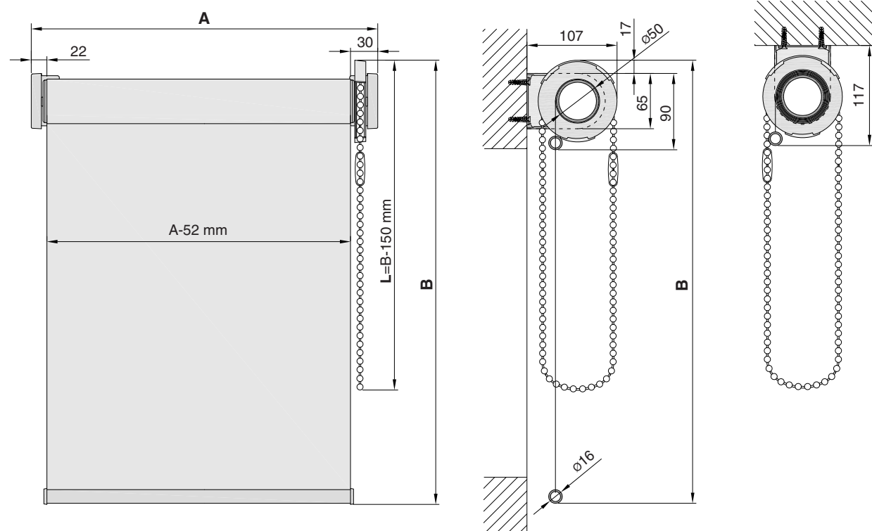
APOLLO PLUS - řetízek
