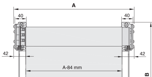
V63 - motor s vedením
