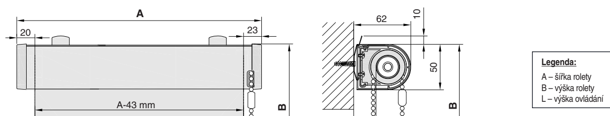
MODULA 25 - PK (s montážním Profilem a Kazetou)
