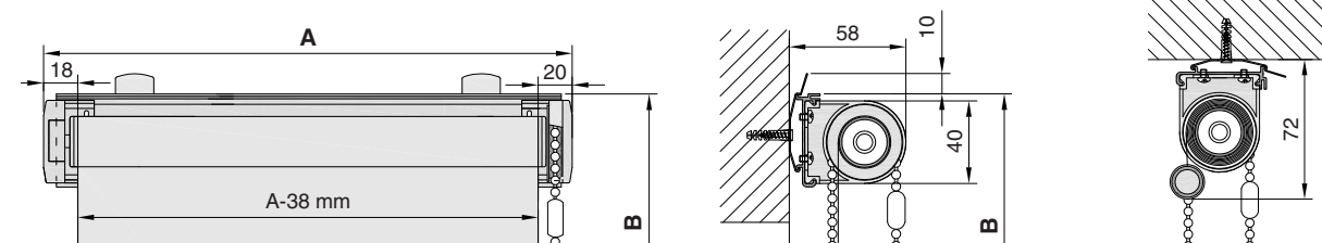
MODULA 25 - P (s montážním Profilem)
