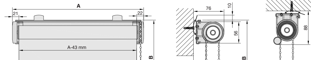
MODULA 36 - P (s montážním Profilem)
