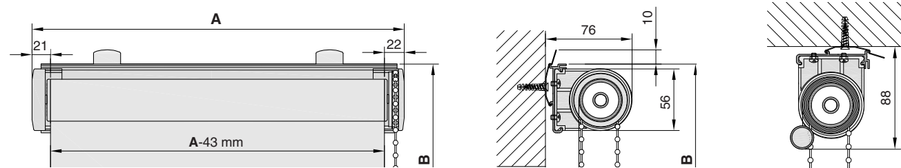
MODULA 38 - P (s montážním Profilem)
