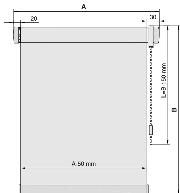
APOLLO - řetízek
