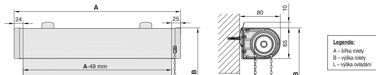
MODULA 38 - PK (s montážním Profilem a Kazetou)
